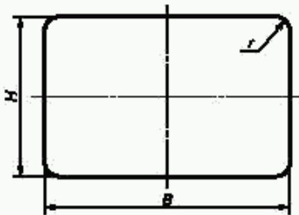
Рисунок Д.8 — Размеры прямоугольных знаков горизонтального формата
