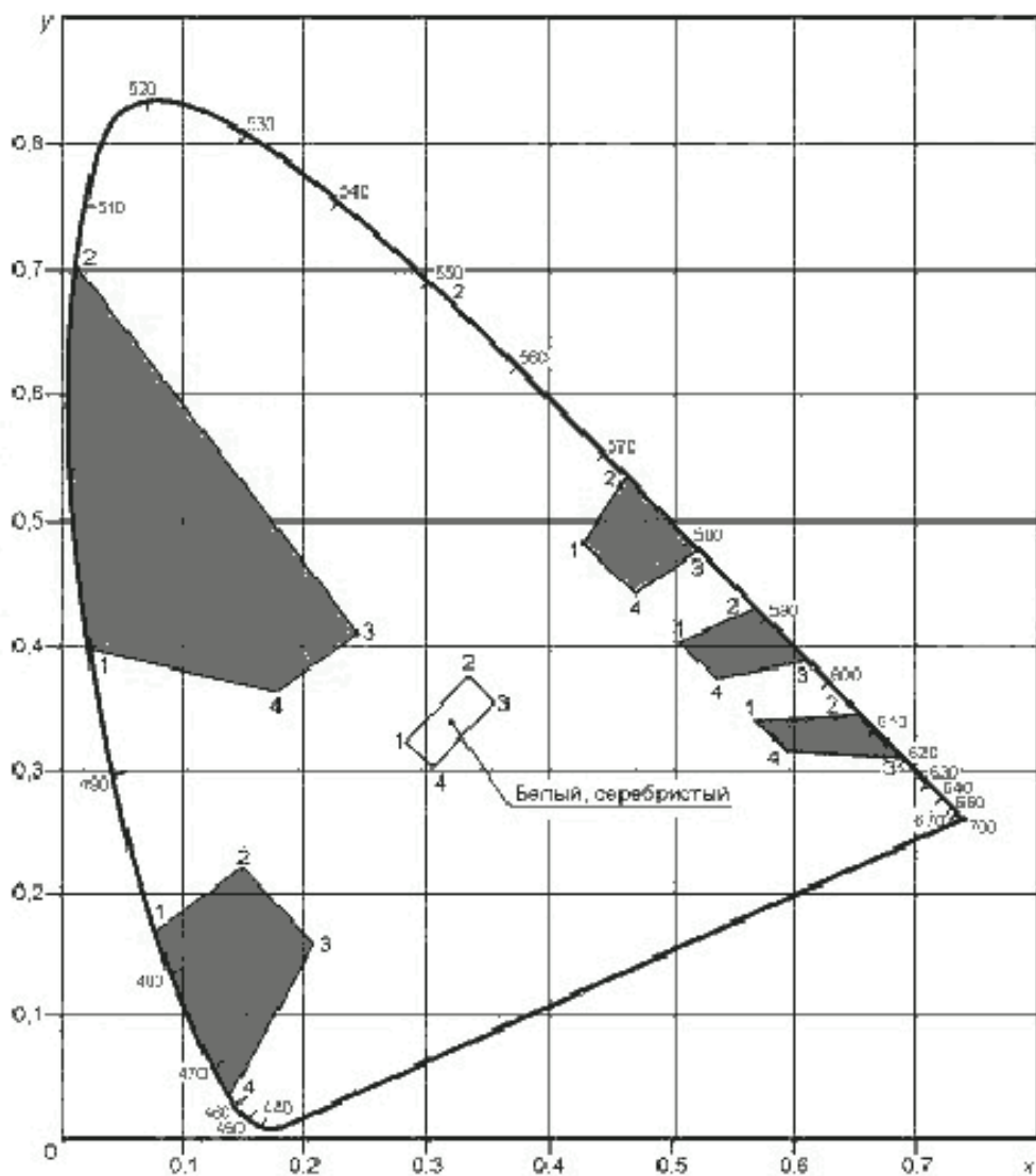
Рисунок 1 — График цветных областей для знаков со светоотражающей поверхностью
