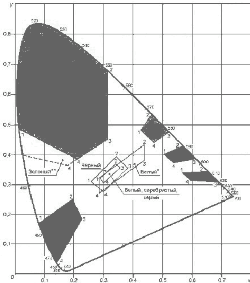
Рисунок 2 — График цветных областей для знаков с внутренним и внешним освещением
